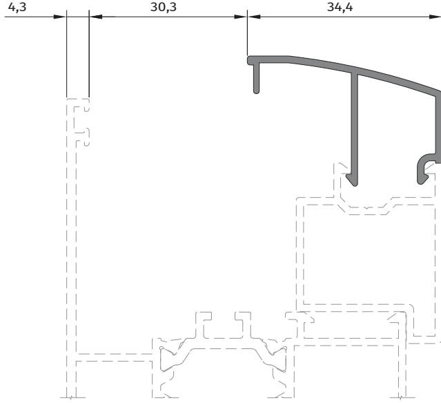
Kasa Detayı / Frame Detail
