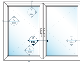
J ORTA KAYITLI 2 KANAT AÇILIR ÜNİTE TWO SASH OPENING + OPENING UNIT W/MIDDLE
