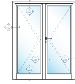
J EŞİKSİZ ÇİFT KANAT DIŞA AÇILIR KAPI WITHOUT SILL DOUBLE OUTSWING DOOR
