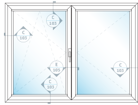
I ÇİFT KANAT ADAPTÖR 2 KANAT AÇILIR + ÇİFT AÇILIM ÜNİTE TWO SASH TILT & TURN + OPENING UNIT W/HIDDEN ADAPTOR
