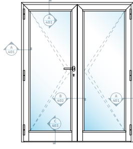
D EŞİKSİZ ÇİFT KANAT İÇE AÇILIR KAPI WITHOUT SILL DOUBLE INSWING DOOR
