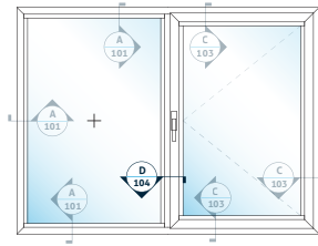
F AÇILIR + SABİT ÜNİTE OPENING + FIXED UNIT
