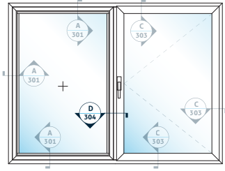
F AÇILIR + SABİT ÜNİTE OPENING + FIXED UNIT
