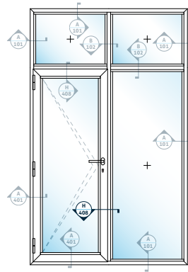
M SABİT + İÇE AÇILIR KAPI FIXED + INSWING DOOR
