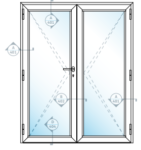
F DÜŞÜK EŞİK ÇİFT KANAT İÇE AÇILIR KAPI LOW SILL DOUBLE INSWING DOOR
