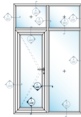
N SABİT + DIŞA AÇILIR KAPI FIXED + OUTSWING DOOR
