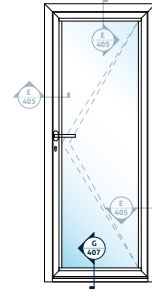
K DÜŞÜK EŞİK TEK KANAT DIŞA AÇILIR KAPI LOW SILL SINGLE OUTSWING DOOR
