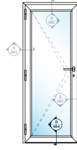
E DÜŞÜK EŞİK TEK KANAT İÇE AÇILIR KAPI LOW SILL SINGLE INSWING DOOR
