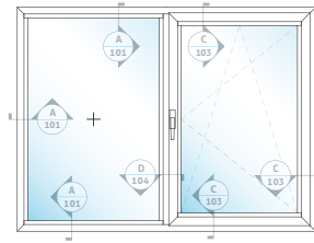
G ÇİFT AÇILIM + SABİT 2 KANAT ÜNİTE TWO SASH TILT & TURN + FIXED UNIT
