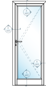
I EŞİKSİZ TEK KANAT DIŞA AÇILIR KAPI WITHOUT SILL SINGLE OUTSWING DOOR
