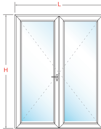
İnce Kasa Çift Kanat Eşiksiz İçe Açılır Kapı Thin Frame Inswing Double Door With Sill Profile
