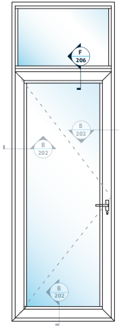
F İNCE KASA İÇE AÇILIR ORTAKAYIT BİRLEŞİMİ THIN SASH INSWING TRANSOM CONNECTION
