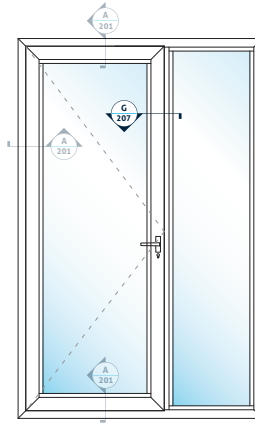
G YAN İÇE AÇILIR ORTAKAYIT BİRLEŞİMİ SIDE INSWING TRANSOM CONNECTION
