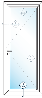
C TEK KANAT DIŞA AÇILIR KAPI SINGLE OUTSWING DOOR
