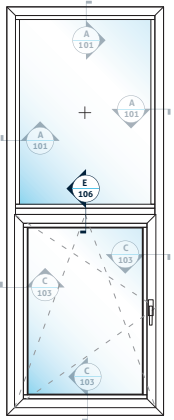
G ORTAKAYIT BİRLEŞİM SABİT+AÇILIR TRANSOM CONNECTION FIX+OPENING
