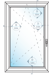
F İNCE KASA ÇİFT AÇILIM 1 PANEL ÜNİTE THIN ONE SASH TILT & TURN UNIT
