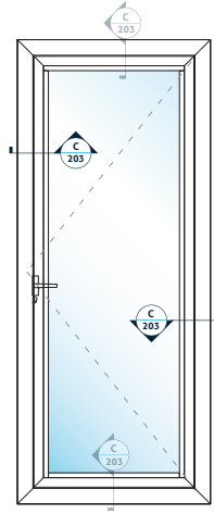
C 203 Tek Kanat Dışa Açılır Kapı Detay Single Outswing Door Detail
