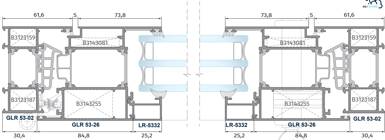
B İnce Kasa Tek Kanat İçe Açılır Kapı Detay 202 Thin Frame Single Inswing Door Detail
