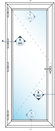
B İnce Kasa Tek Kanat İçe Açılır Kapı Detay 202 Thin Frame Single Inswing Door Detail
