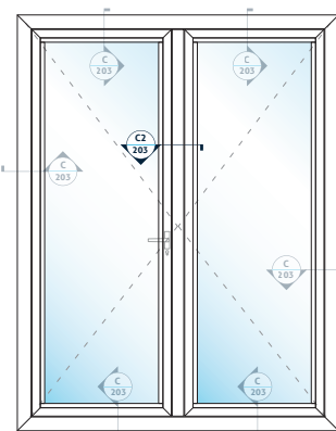
C2 DIŞA AÇILIR ÇİFT KANAT KAPI OUTSWING DOUBLE DOOR
