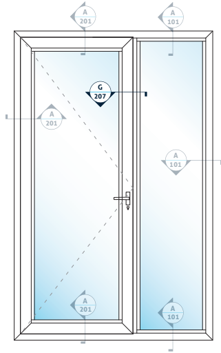
G 207 Yan Birleşim Ortakayıt İçe Açılır Side Connection Transom Inswing
