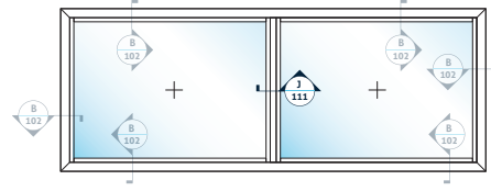
J 111 İnce Kasa Sabit + Sabit Ortakayıt Birleşim Thin Sash Fix +Fix Transom Connection
