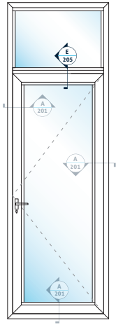
E İÇE AÇILIR ORTAKAYIT BİRLEŞİMİ INSWING TRANSOM CONNECTION
