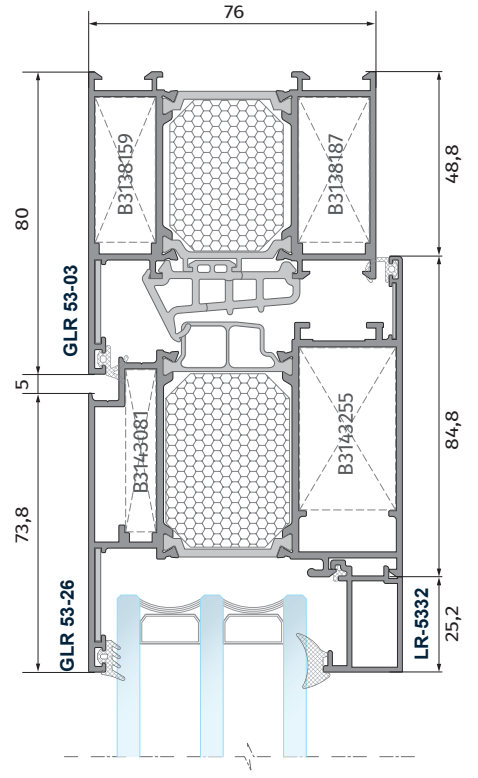
A 201 Tek Kanat İçe Açılır Kapı Detay Single Inswing Door Detail
