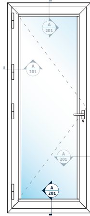
A 201 Tek Kanat İçe Açılır Kapı Detay Single Inswing Door Detail
