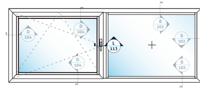
L 113 İnce Kasa Açılır Panel + Sabit Ortakayıt Birleşim Thin Sash Opening Panel +Fix Transom Connection
