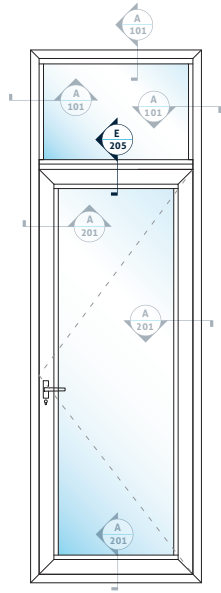
E 205 Dışa Açılır Ortakayıt Birleşim Outswing Transom Connection
