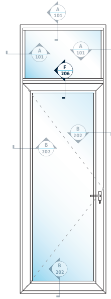
F 206 İçe Açılır Ortakayıt Birleşim Inswing Transom Connection
