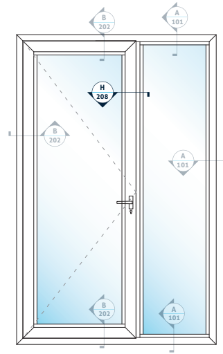
H 208 Yan Birleşim Ortakayıt İçe Açılır İnce Kasa Side Connection Transom Inswing Thin Sash
