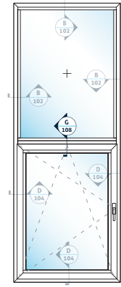
I İNCE KASA BİRLEŞİM SABİT+AÇILIR THIN SASH CONNECTION FIX + OPENING
