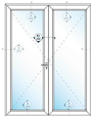
B2 İNCE KASA ÇİFT KANAT İÇE AÇILIR KAPI THIN FRAME INSWING DOUBLE DOOR
