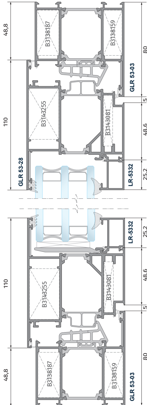
C 203 Tek Kanat Dışa Açılır Kapı Detay Single Outswing Door Detail
