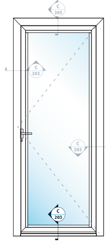
C 203 Tek Kanat Dışa Açılır Kapı Detay Single Outswing Door Detail
