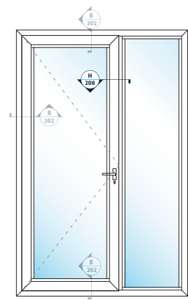
H İNCE KASA YAN İÇE AÇILIR ORTAKAYIT BİRLEŞİMİ SIDE THIN SASH INSWING TRANSOM CONNECTION
