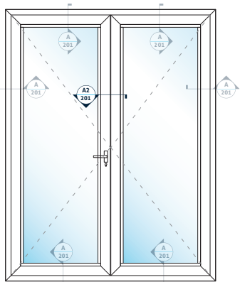
A2 İÇE AÇILIR ÇİFT KANAT KAPI INSWING DOUBLE DOOR
