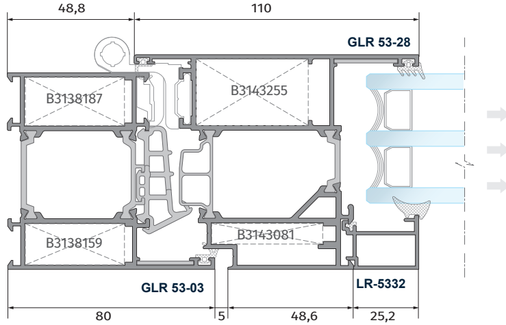
C2 Dışa Açılır Çift Kanat Kapı 203 Outswing Double Door
