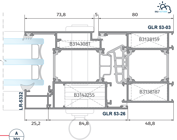
A Tek Kanat İçe Açılır Kapı Detay 201 Single Inswing Door Detail
